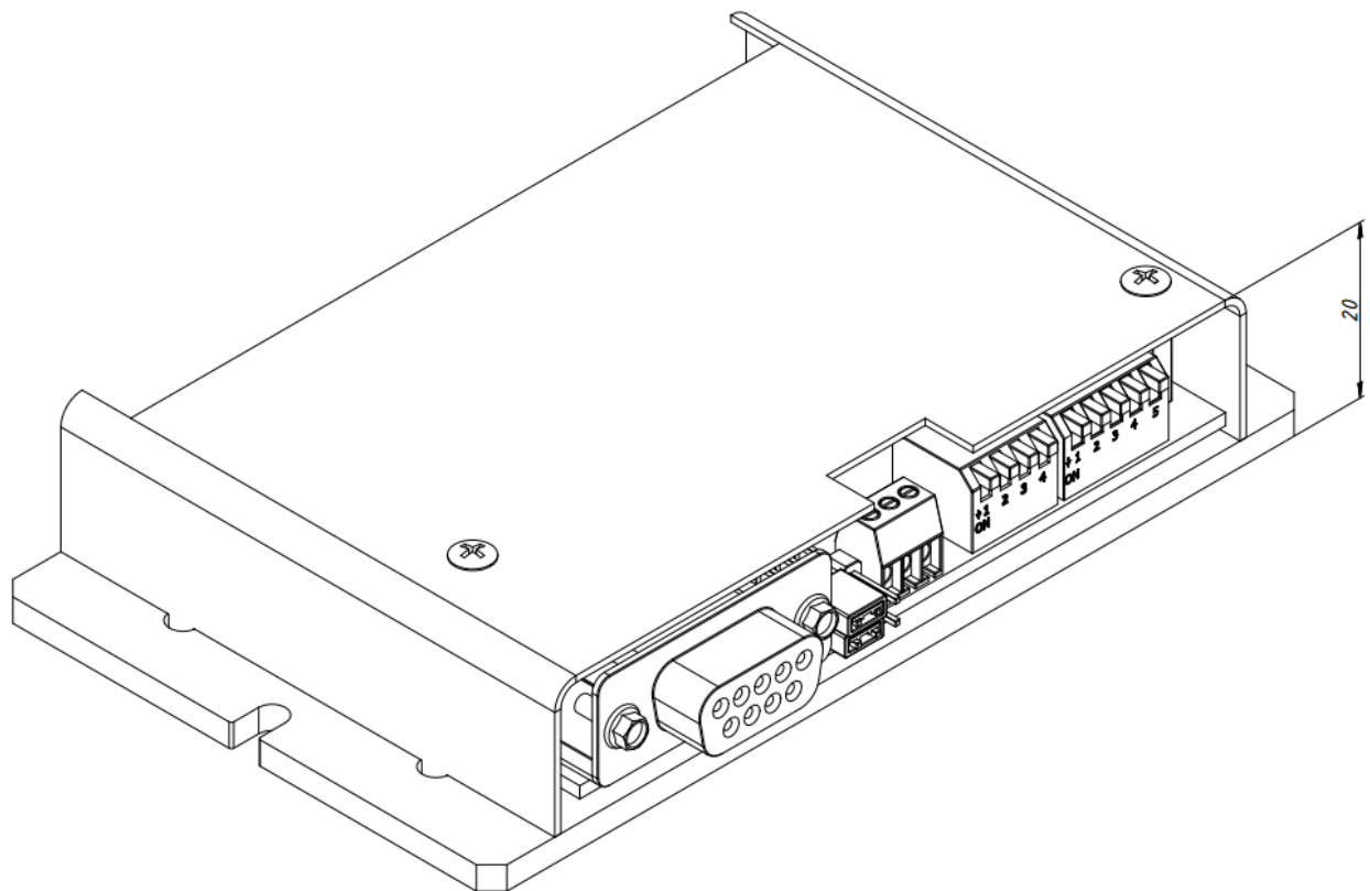
Рисунок 1.2 - Габаритные и присоединительные размеры устройства
